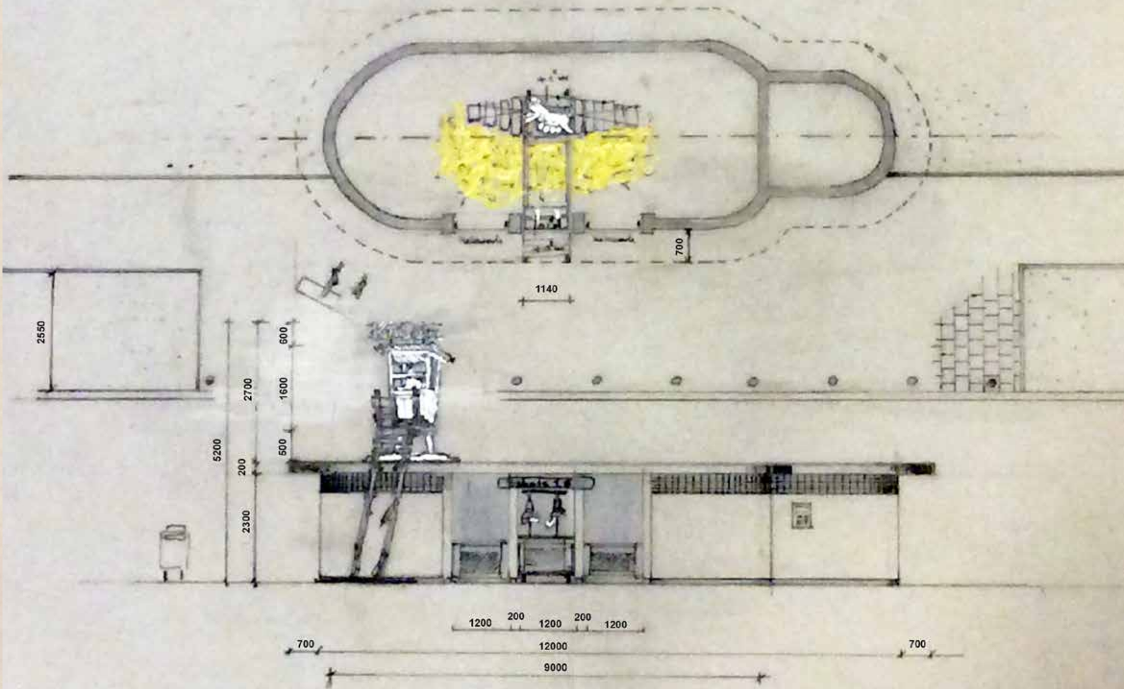
Vooraanzicht Schreiershuisje met installatie in en op het gebouw.
